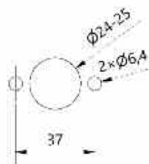
vrtání otvorů pro MG rozety
