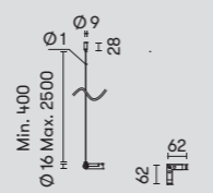
71-8259-05-05 ■ 90° horizontal connector | Conector 90° horizontal | Connecteur 90° horizontal
