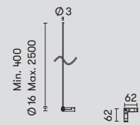
71-8254-05-05 ■ 90° horizontal connector | Conector 90° horizontal | Connecteur 90° horizontal
